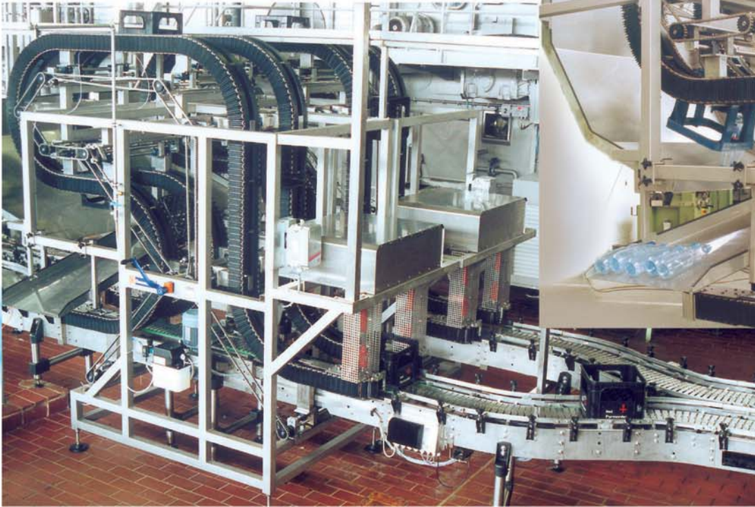
Deckelbenetzer für die Kalt- und Heissabfüllung von Softdrinks wie Fruchtsaft usw. Eine einfache und kostengünstige Lösung um Flaschen zum Zwecke der Kopfraumbenetzung zu kippen oder zu wenden. Durch unterschiedliche Bauformen können die Anlagen direkt in die Linie integriert oder als Bypass-Lösung eingebunden werden.
